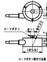
ロードボタン取付寸法図
