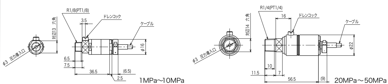
■外形寸法図 (単位：mm)
