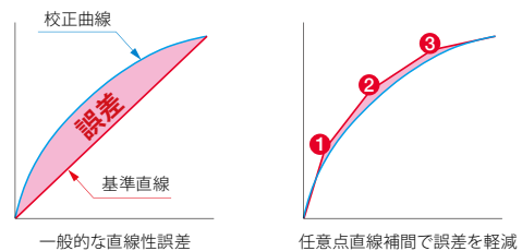
一般的な直線性誤差
