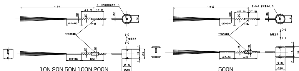
■外形寸法図 (単位：mm) ※詳細はwebサイトをご参照ください。
