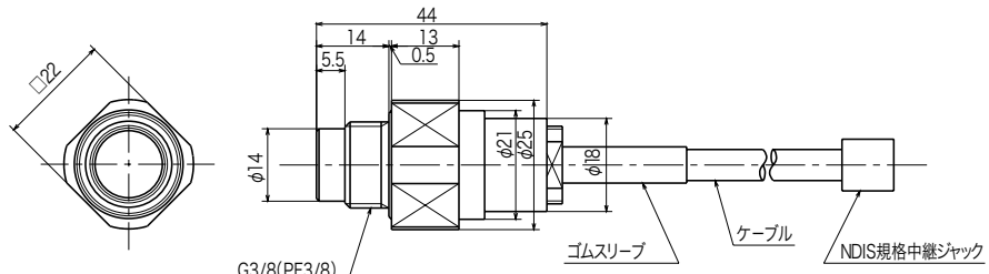
■外形寸法図 (単位：mm)
