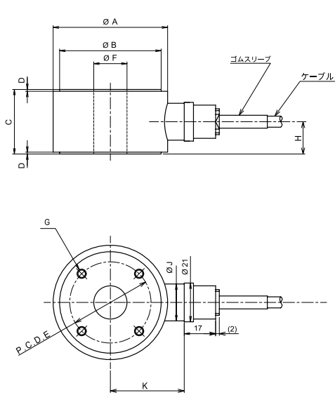
■外形寸法図 (単位: mm)
