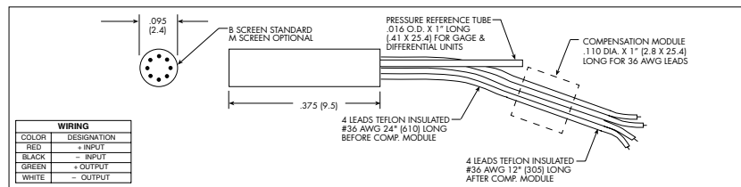
■ 外形寸法図 単位: インチ (※カッコ内: mm)
