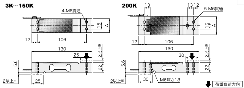
■外形寸法図 (単位: mm)
