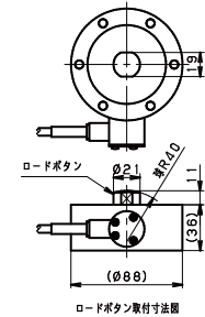
ロードボタン取付寸法図
