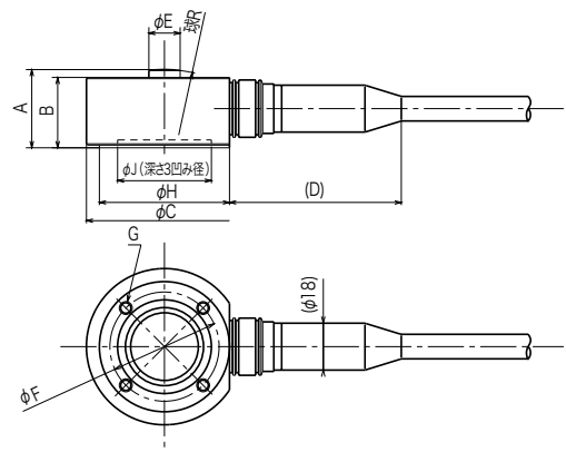
■外形寸法図 (単位: mm)
